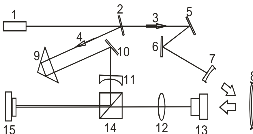
Рис. 2. Схема записи голограмм для измерения наноперемещений
