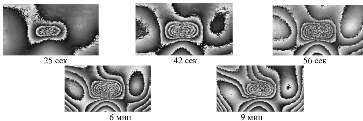
8-расм. Объект сиртидаги қизиш динамикасини кўрсатувчи интерферограммалар
