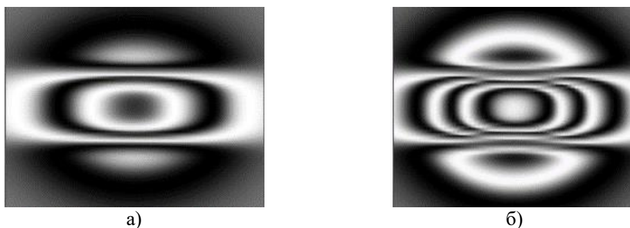
Рис.10. Расчет фоторефрактивной структуры в кристалле \text{LiNbO}_3:\text{Fe}
