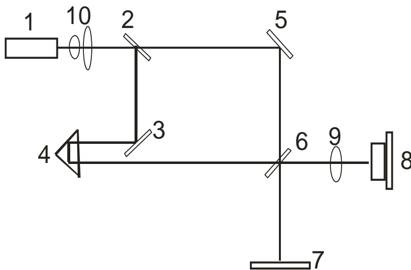
1 – импульс лазери; 2, 6 – ёруғлик бўлувчи пластиналар; 3, 5 – кўзгу; 4 – кечиктириш йўли; 7 – тадқиқот олиб борилаётган объект; 8 – ПЗС матрица; 9 – йиғувчи линза; 10 – телескопик тизим
