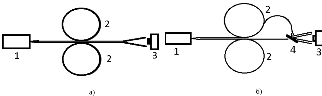
1 – лазер, 2 – оптик тола, 3 – рақамли камера, 4 – ёруғликни бўлувчи пластина 1-расм. Юнг ва Майкельсон интерферометрлари асосида йиғилган ўлчов схемалари
