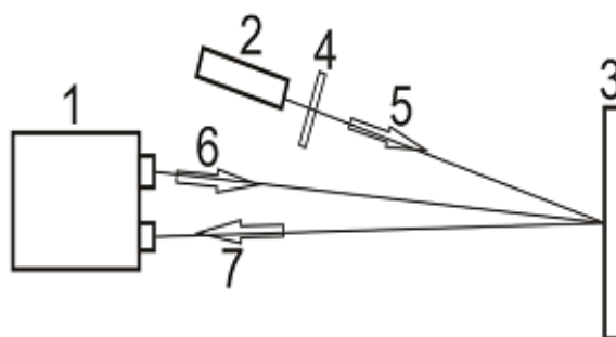
1-интерферометр. 2 – нагревающий лазер. 3 – объект. 4 – светофильтр. 5 – нагревающее излучение. 6 - освещение объекта. 7 – излучение, отраженное от объекта.
