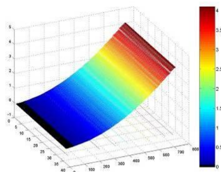
Рис. 6. Результаты измерения прогибов модельной балки
