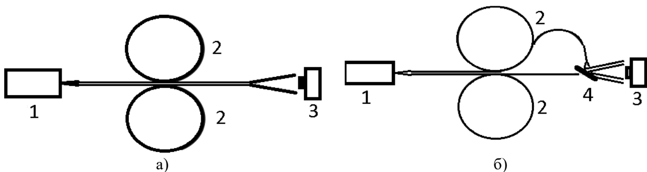
Рис. 1. Схемы измерений, основанные на интерферометре Юнга и Майкельсона
