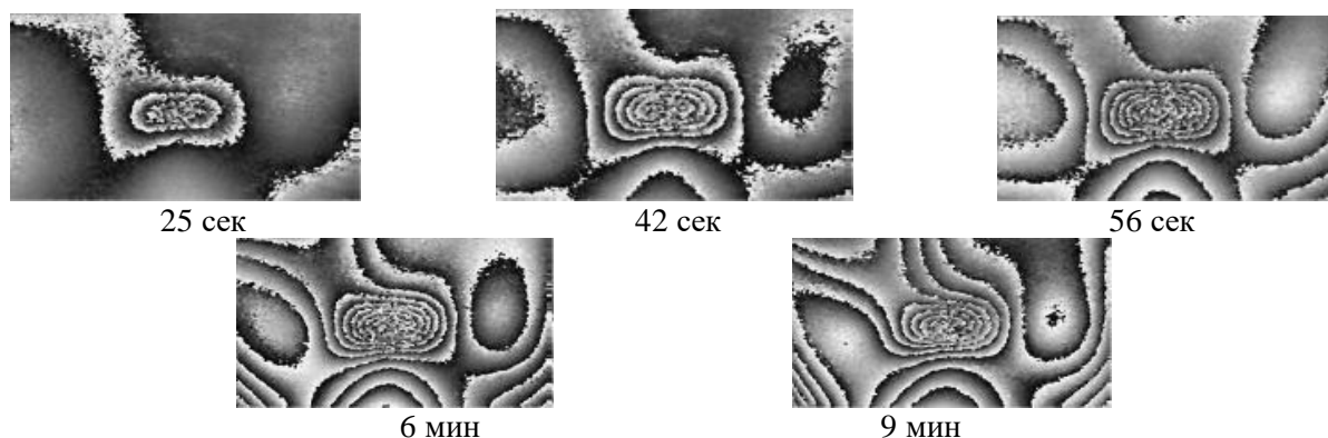
Рис. 8. Интерферограммы, отражающие динамику нагрева поверхности объекта
