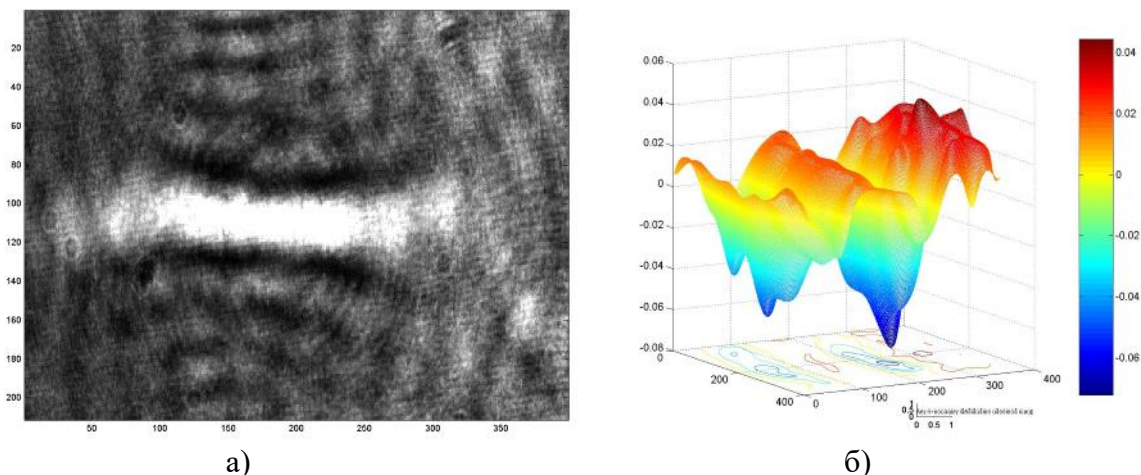
Рис. 11. Интерферограмма и фазовая реконструкция фоторефрактивной структуры
