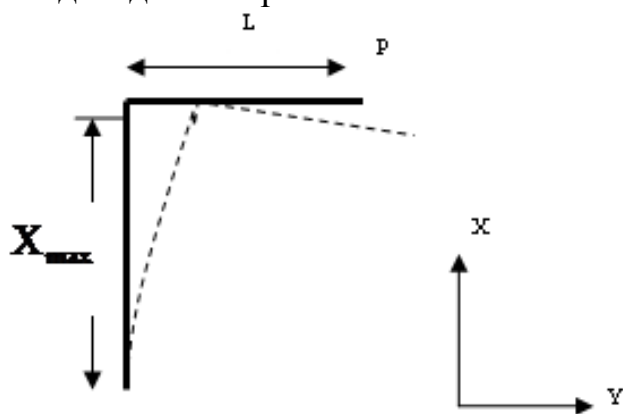
5-расм. Макет балкасига осилган Р юкнинг схемаси
