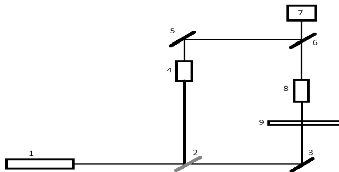
1 – лазер; 2, 6 – оптик пона, 3, 5 – кўзгу; 4, 8 – объектив; 7 – CCD камера, 9 – кремний пластинаси 4-расм. Интроскопнинг оптик схемаси
